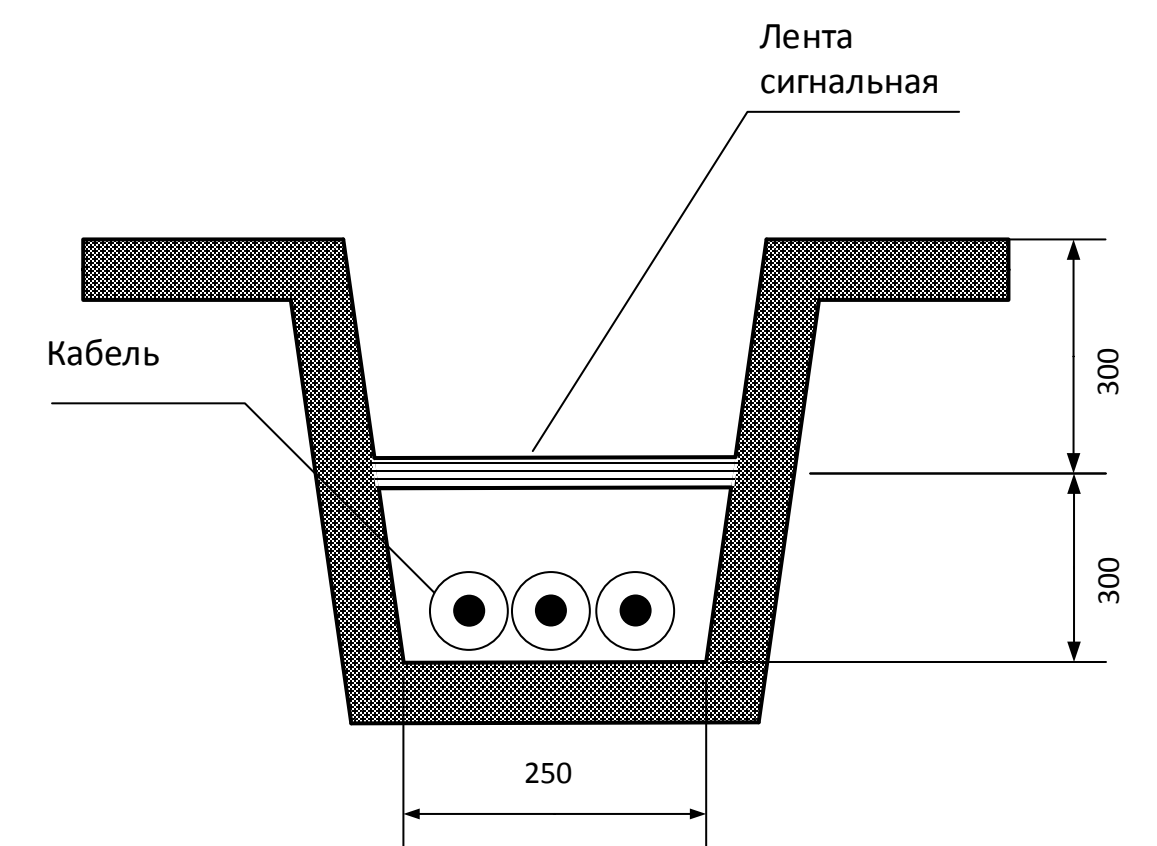
Способ устройства траншеи для кабеленесущих трасс
