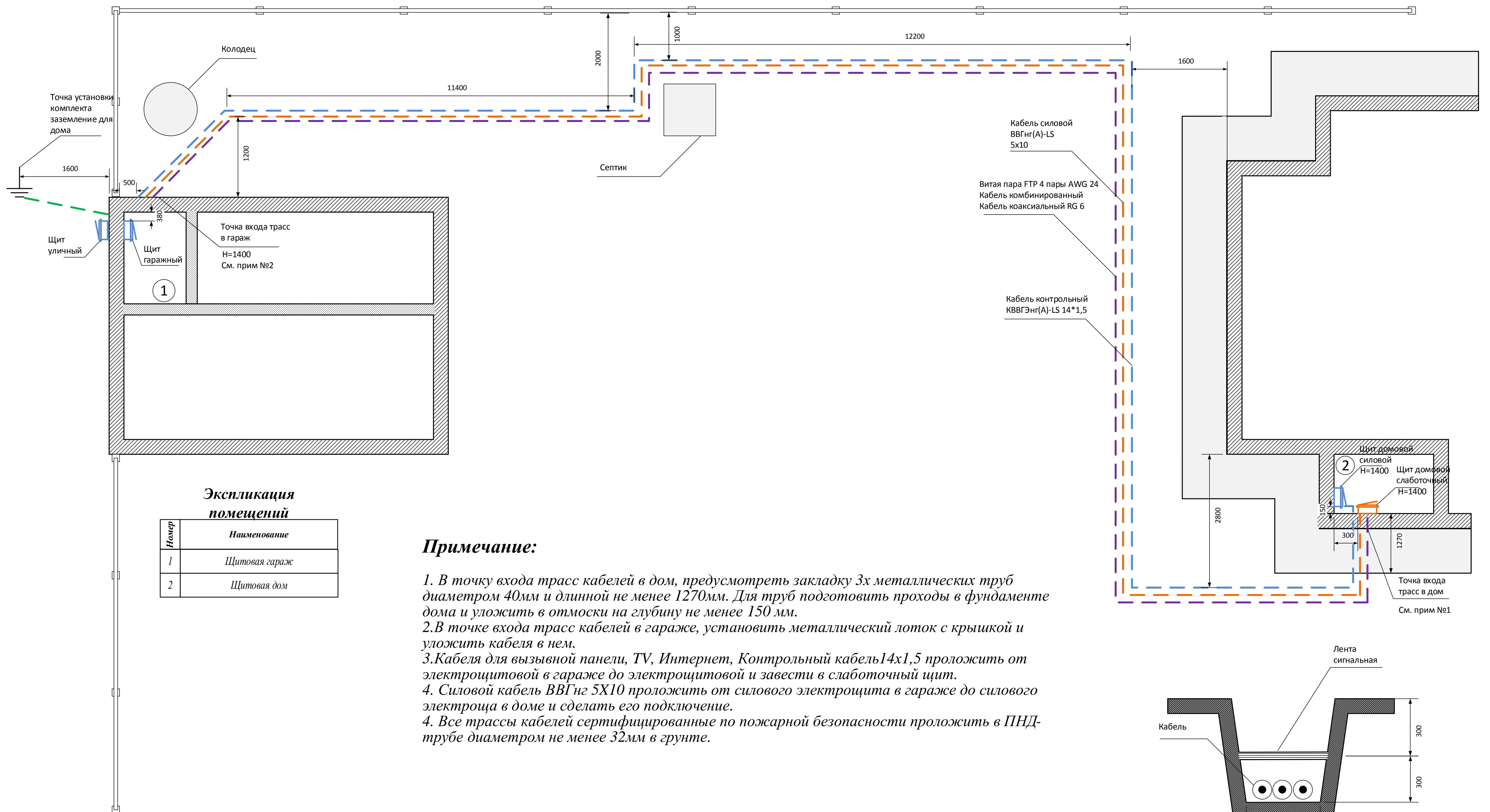
Способ устройства траншеи для кабеленесущих трасс
